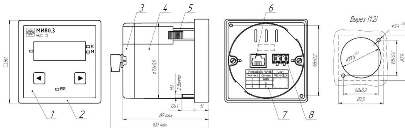
б) модуль МИ80.3
