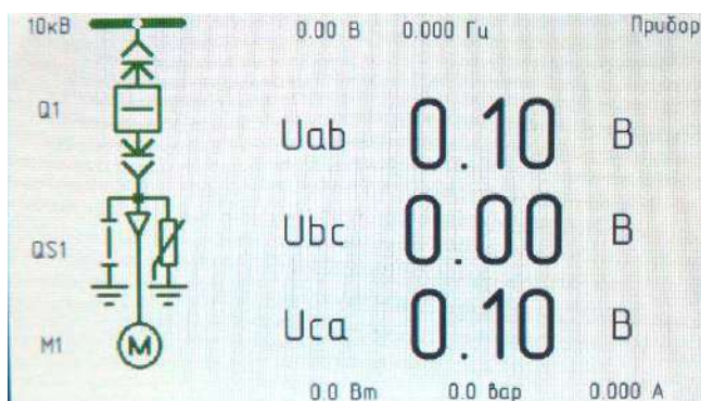
г) мнемосхема
