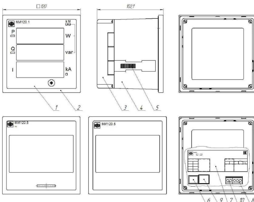
а) модули МИ120.б
