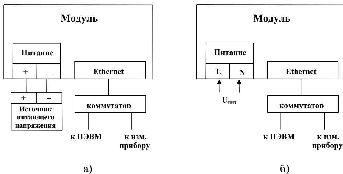
Рисунок Б.3 – Схемы подключения модуля МИ120.5 к измерительному прибору, преобразователю, ПЭВМ по интерфейсу Ethernet на прямую.
